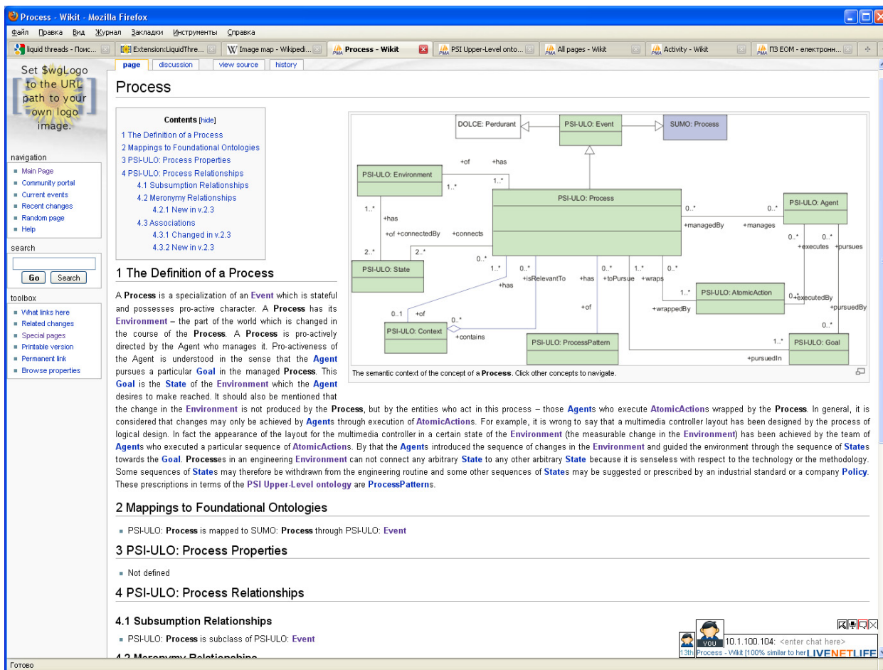
Рис. 1. Wiki страница онлайн документации онтологии верхнего уровня PSI – определение концепта Process
